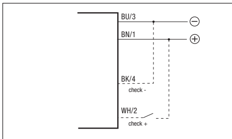
BX04 – BX10 Emettitore / Emitter
