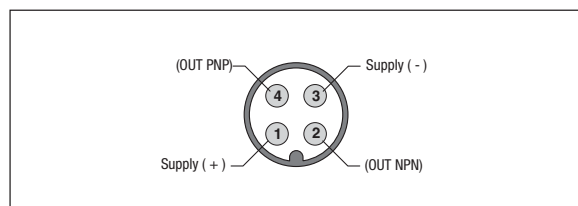
BX04 – BX10 Ricevitore / Receiver
