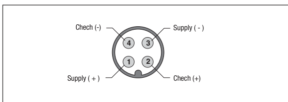
BX04 – BX10 Emittitore / Emitter
